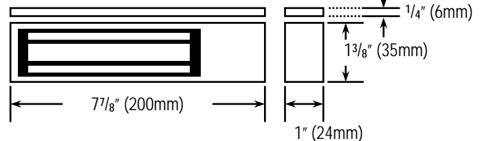
Placa de armadura (para E-941SA-300 y E-941SA-300RQ)
