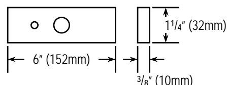
Placa de armadura (para E-941SA-300 y E-941SA-300RQ)
