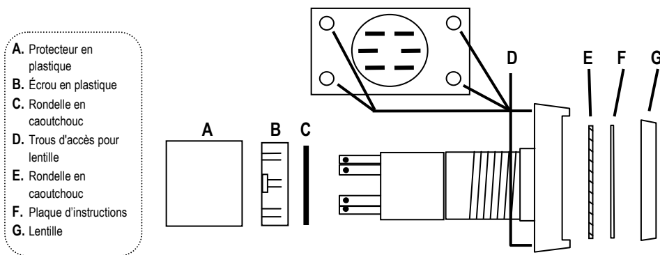
Figure 3 – Sortie minuterie
