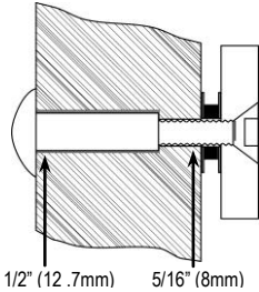
Solid Core Door
