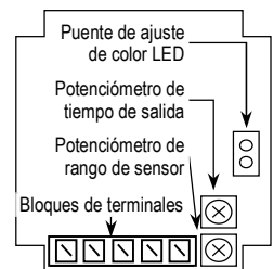
Fig.3 Configuración del puente LED
