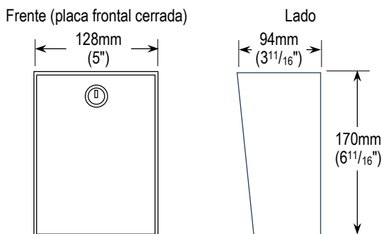
BP-601 mostrado, BP-611 Mismo tamaño y forma
