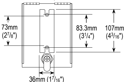
BP-611 Tamaño de la abertura, mostrado desde el interior al abrirse
